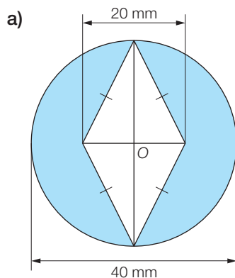
Cercle de centre O
