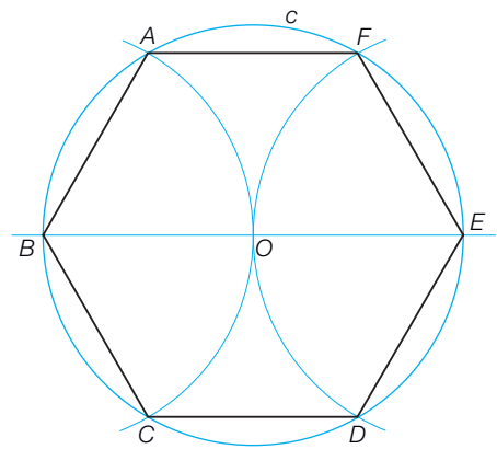
a) Hexagone régulier
